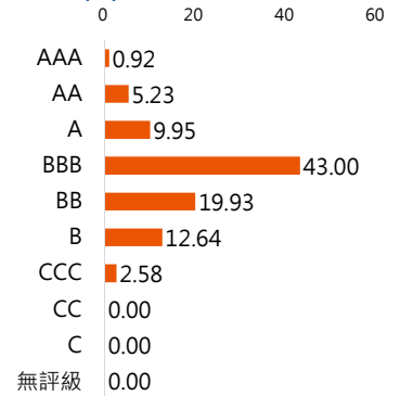
信評分布(%)
