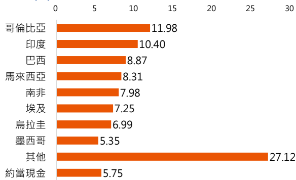
投資國家(%)
