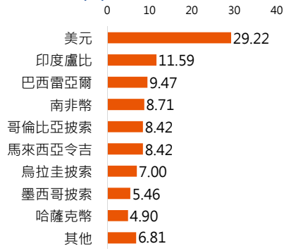
幣別分布(%)
